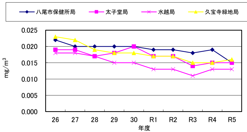
浮遊粒子状物質(SPM) 年平均値 経年変化
