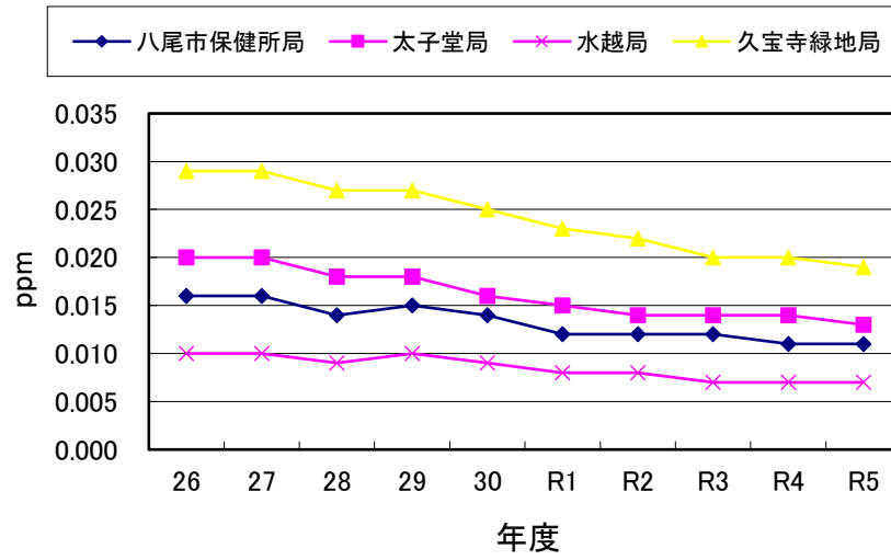
二酸化窒素 年平均値 経年変化
