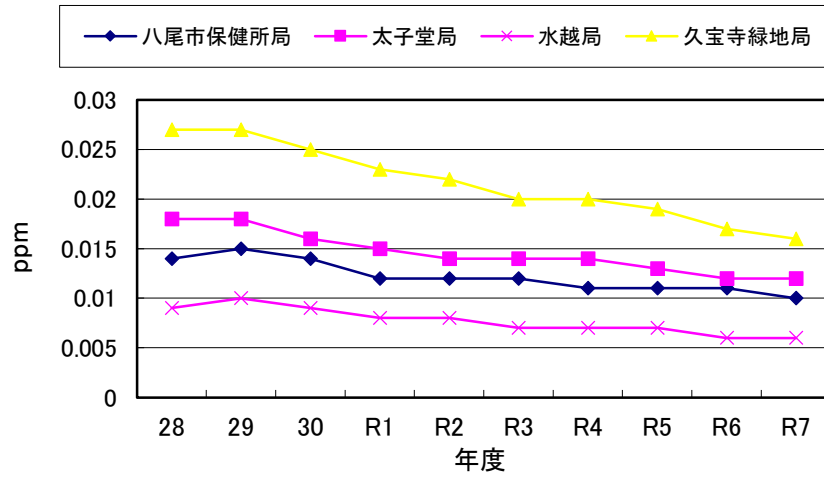
二酸化窒素 年平均値 経年変化
