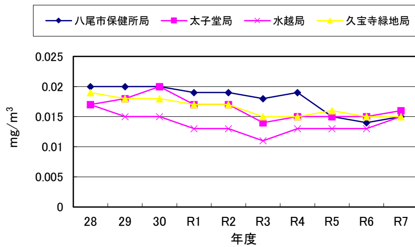
浮遊粒子状物質(SPM) 年平均値 経年変化
