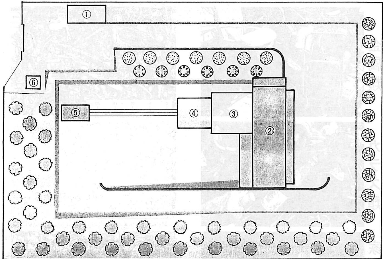
①管理棟 ②貯溜棟 ③破碎棟 ④磁選棟 ⑤貯蔵棟 ⑥倉庫
