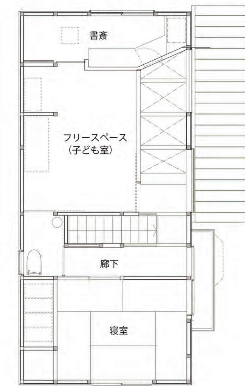
2階平面図
