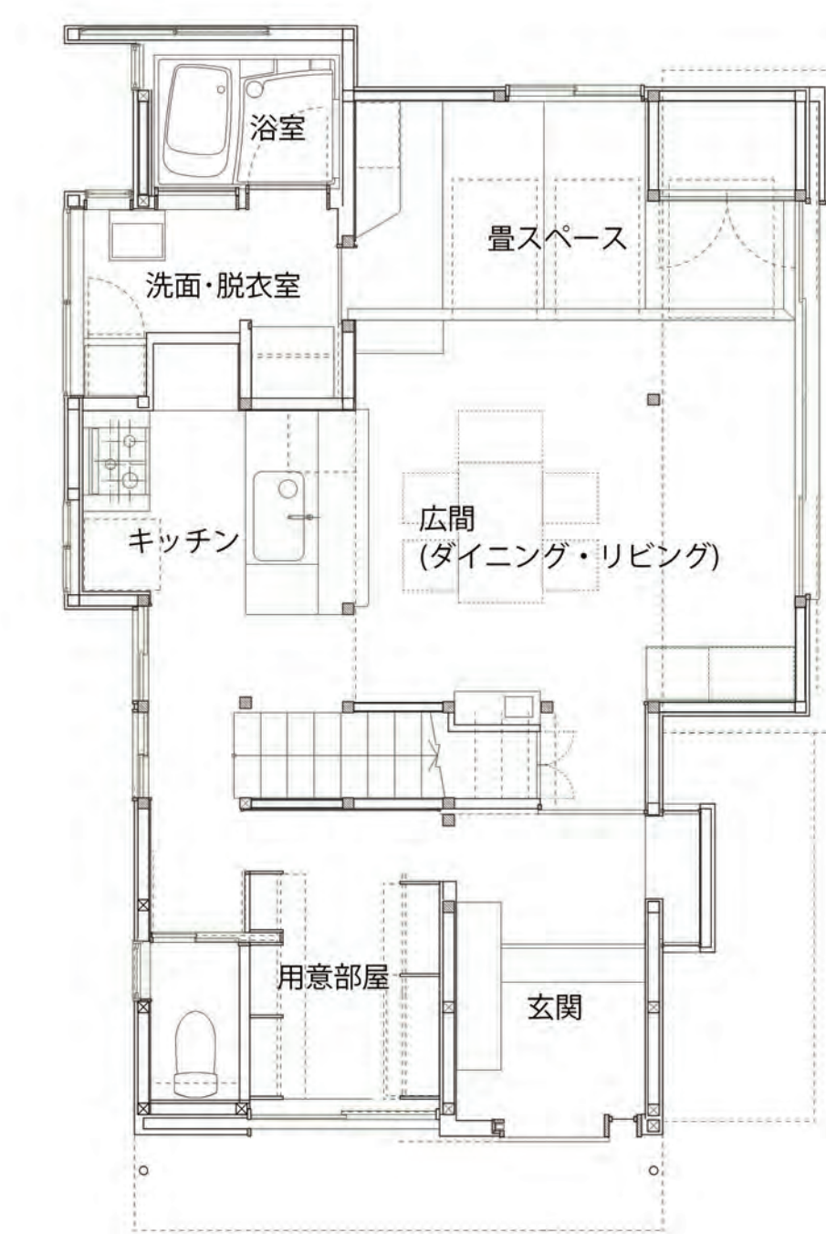
1階平面図
