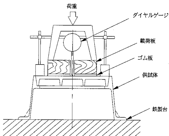
図-2 荷重載荷試験方法
