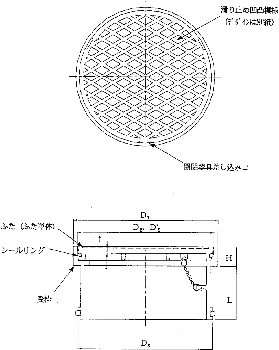
図-2 差し口形ワタチふた (シーリング接合) (略号 A1-R)
