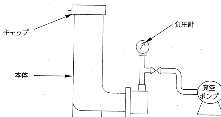
図-3 負圧試験
