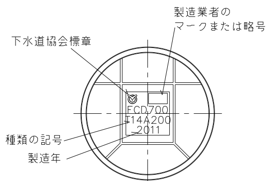
図-3 下水道協会標章及び種類の記号鑄出配置図
