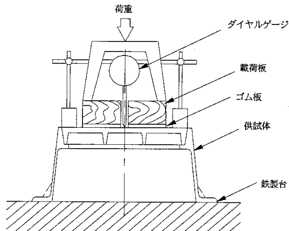
図-2 荷重載荷試験方法
