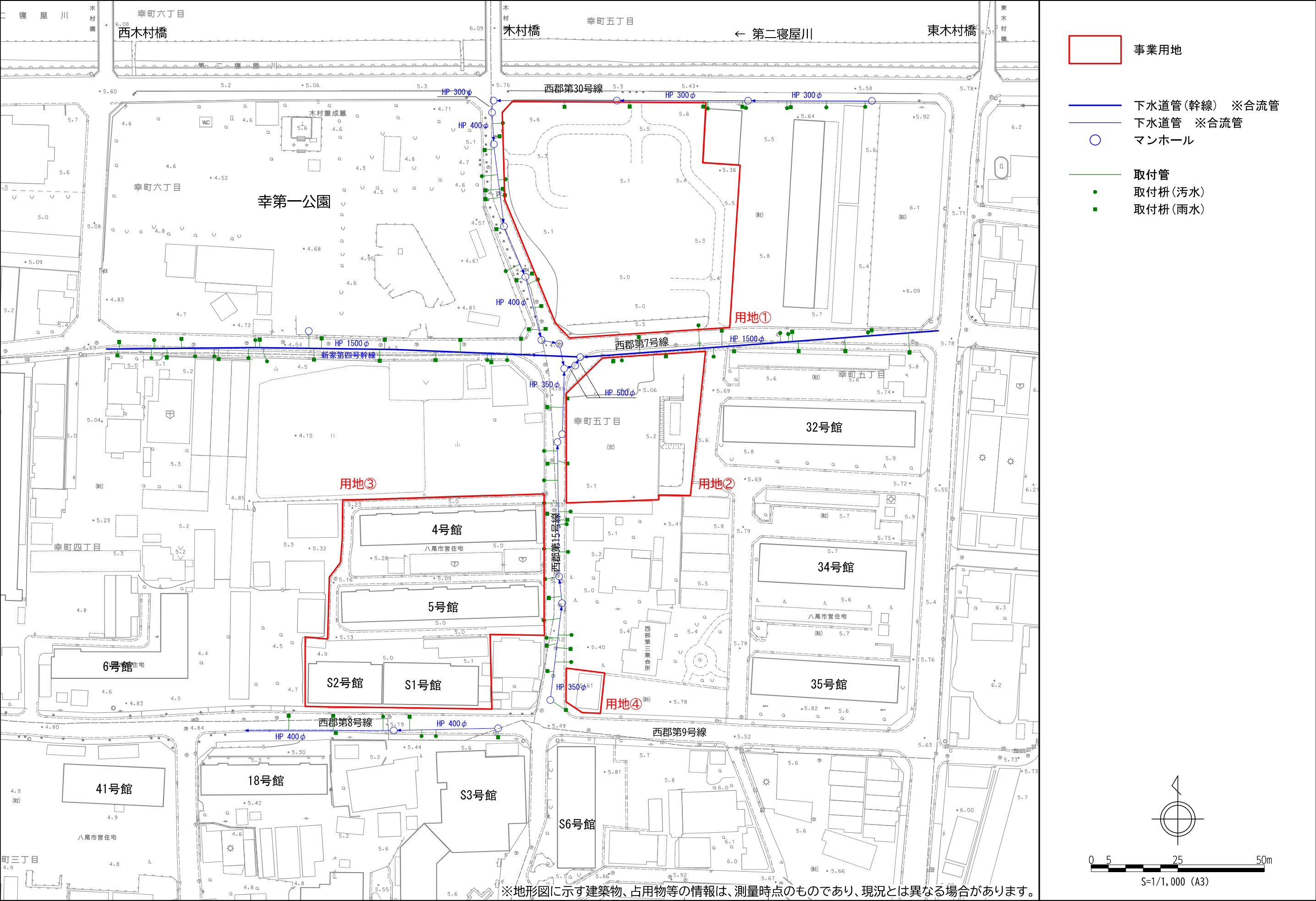
資料5－3 下水道管布設現況図
