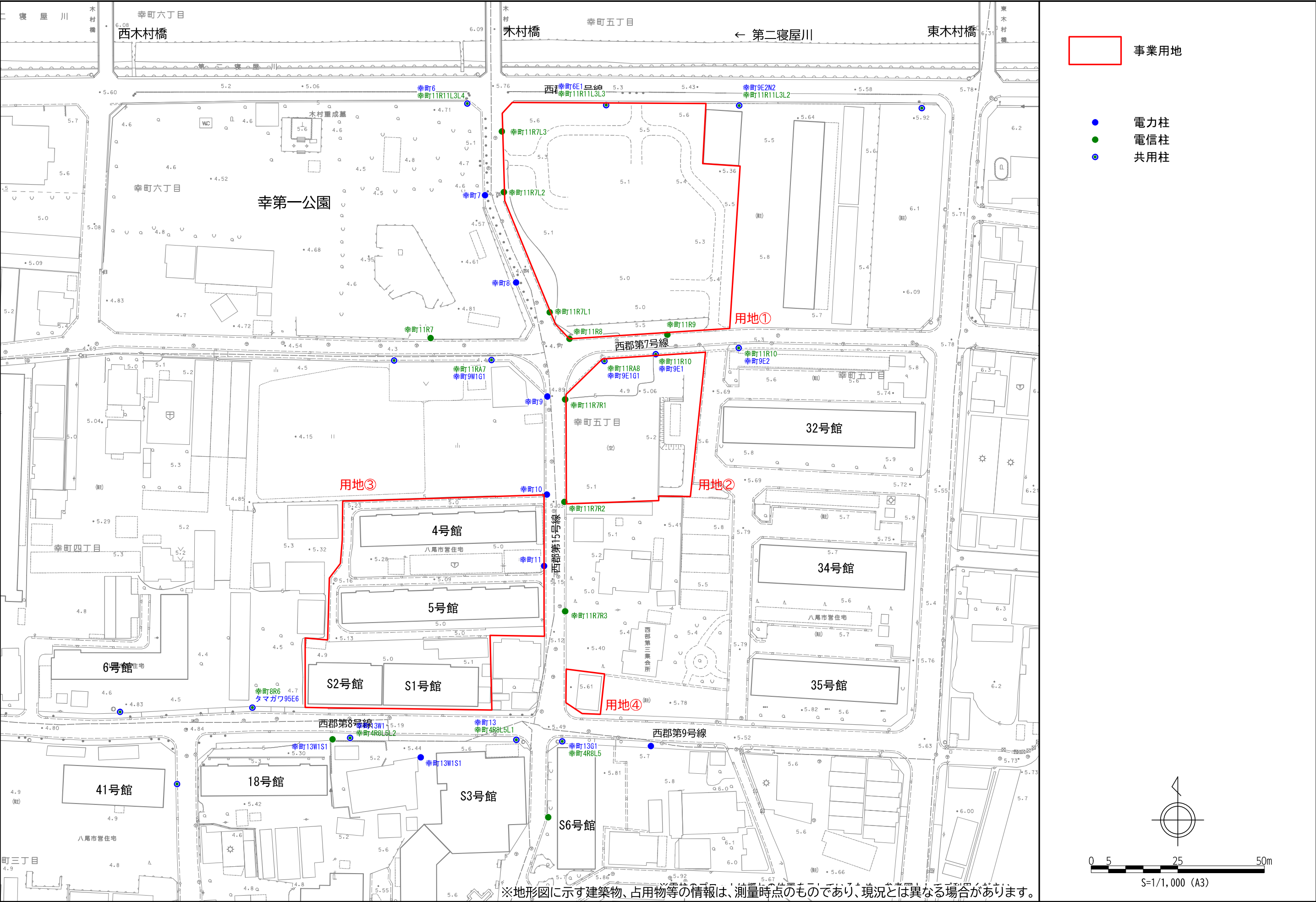
資料 5－5 電柱等設置現況図
