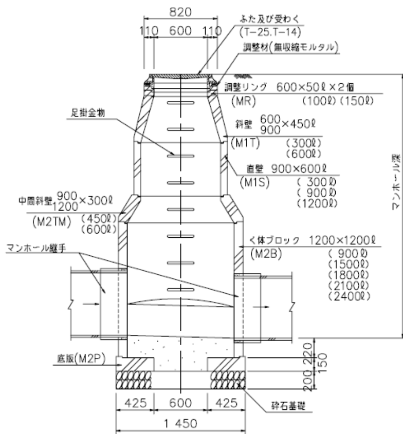
縦断面図
