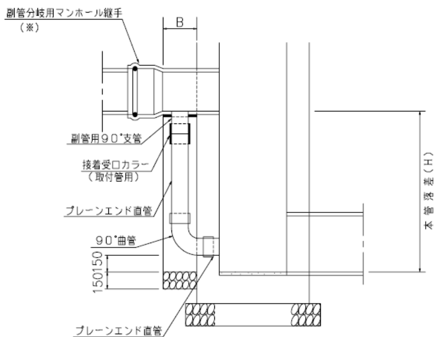
断面図
