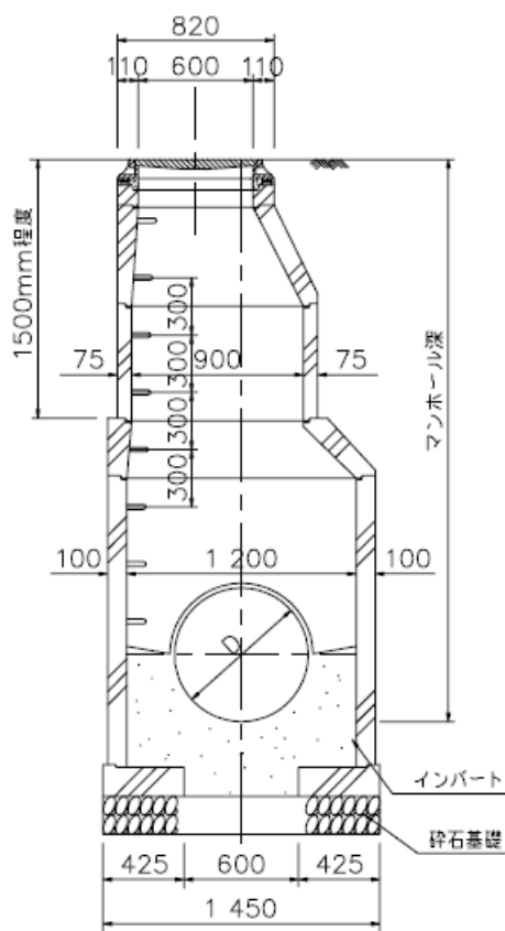
横断面図
