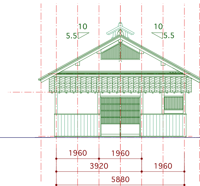
南立面図 1/100
