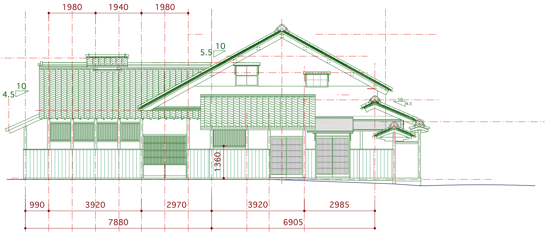
東立面図 1/100
