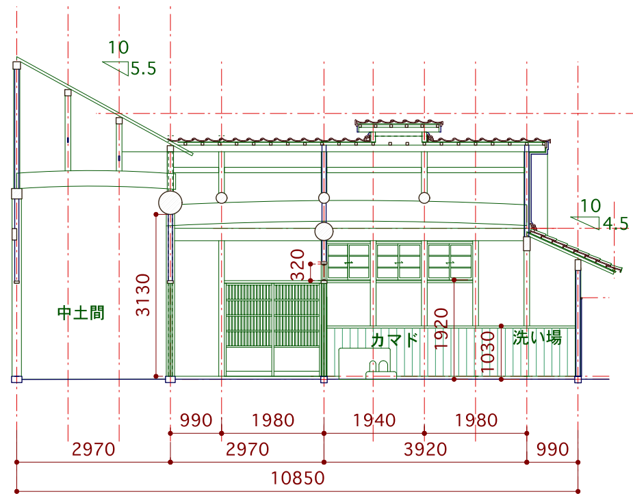
断面図 1/100
