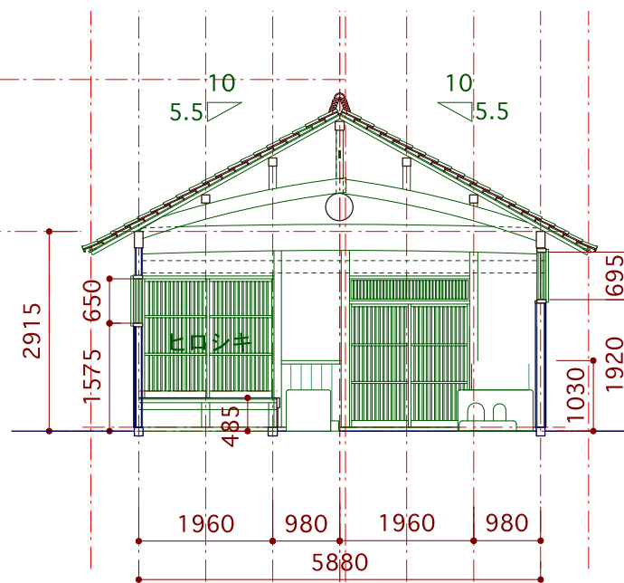
断面図 1/100
