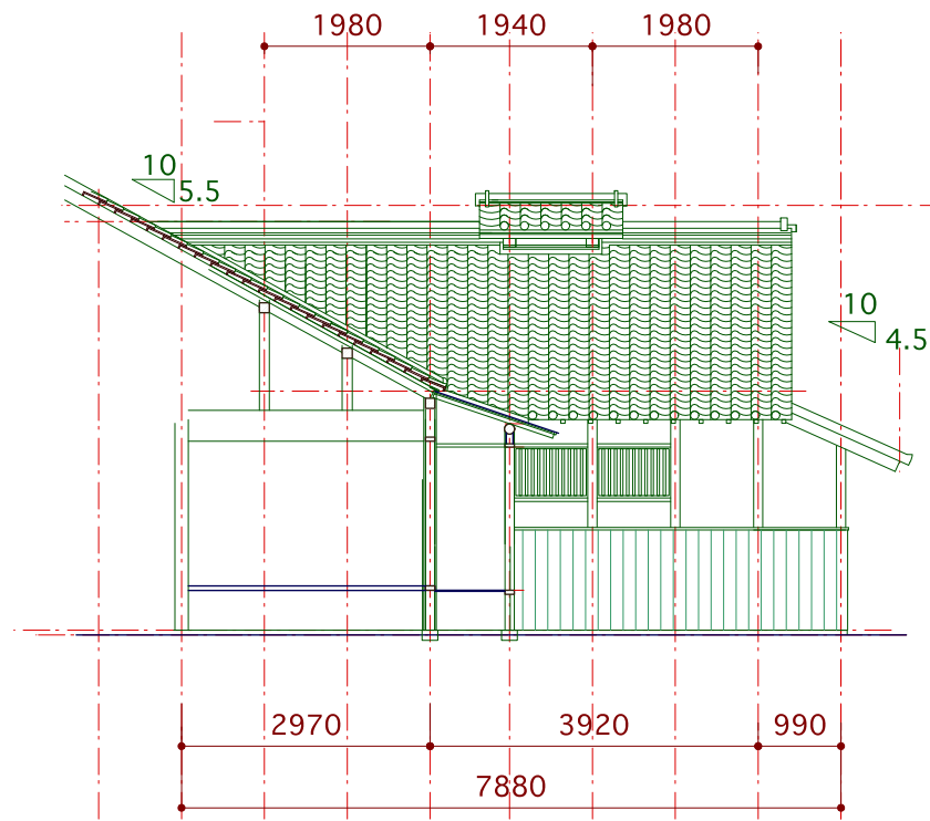
西立面図 1/100
