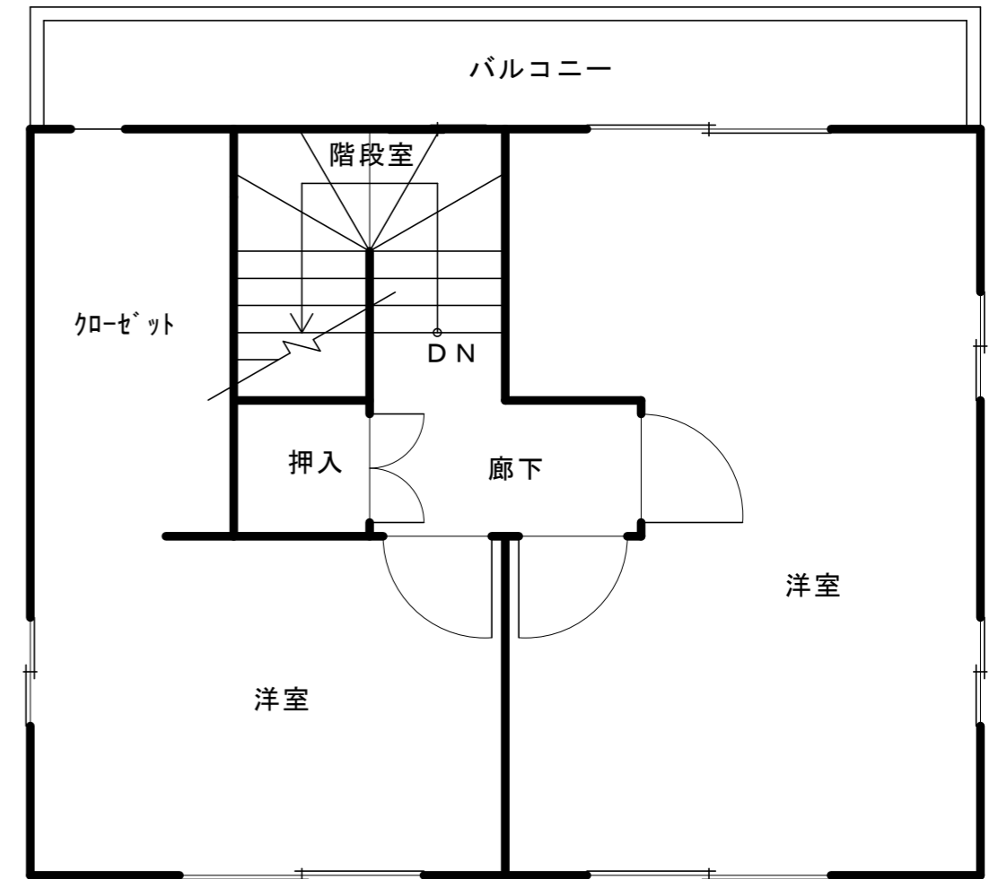
3階平面図
