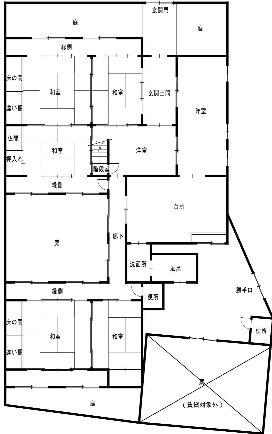
1階平面図
