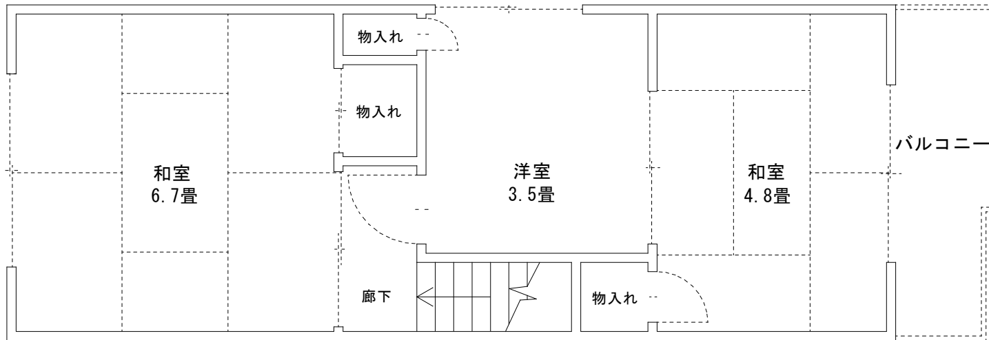
2階平面図
