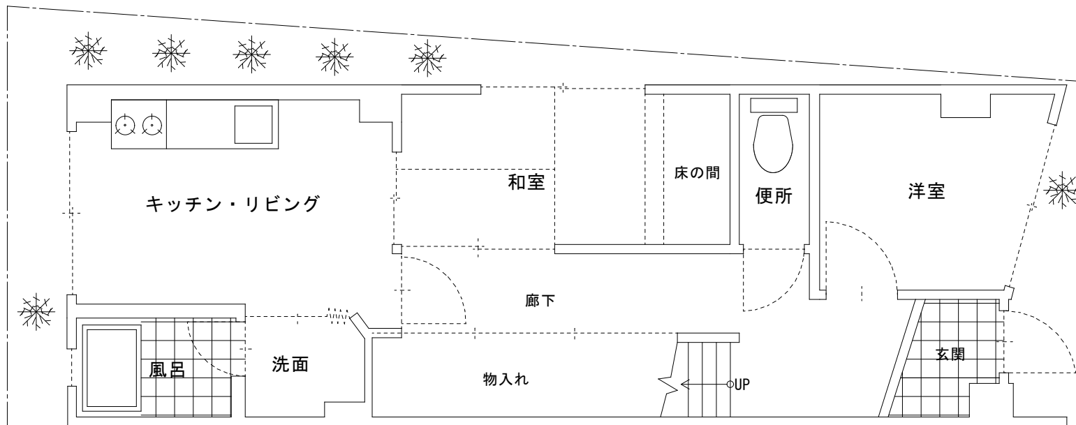
1階平面図・配置図
